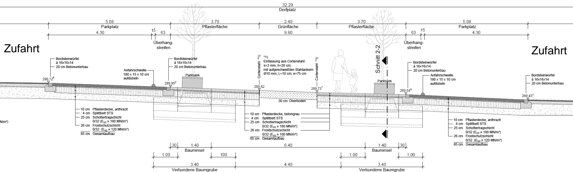
Schnitt 1-1
